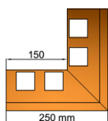
PAL-E 90Z
