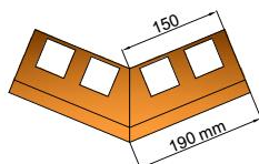
PAL-E 135Z
