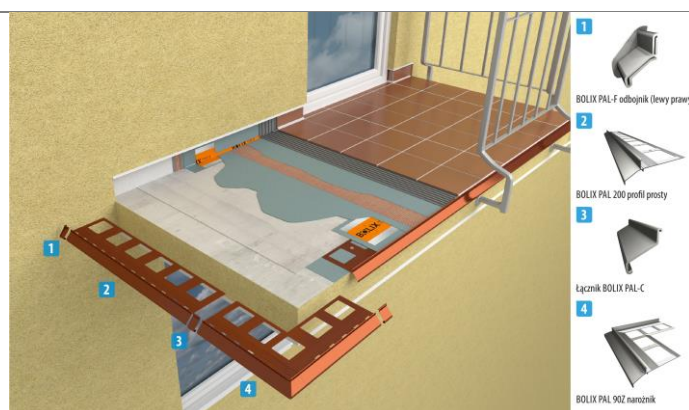
Przekrój poprzeczny przez profil BOLIX PAL 200
